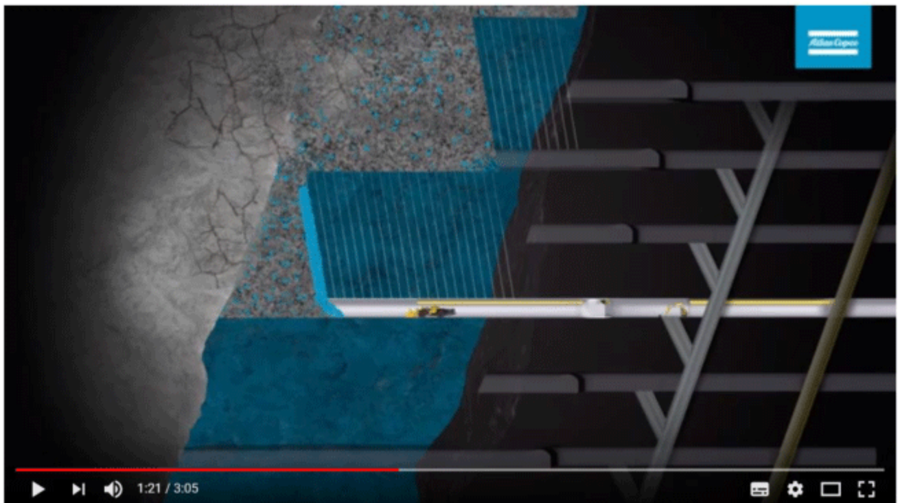
Sublevel Caving Mining Method
